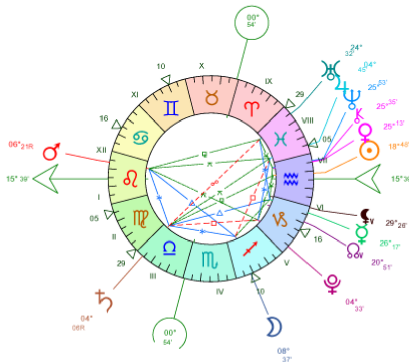
3 e retour de Neptune 7 février 2010 à 13h35 TU à Paris
