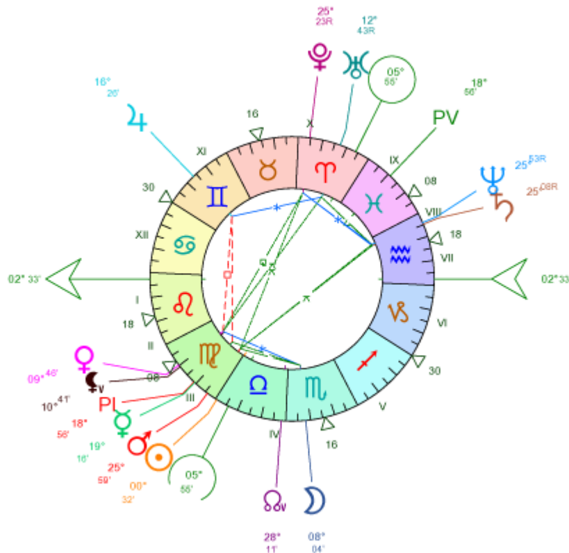
Découverte de Neptune 23 septembre 1846 à 23h30 TU à Berlin
